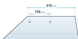
Lemken - Ojačani raonik 3352231
