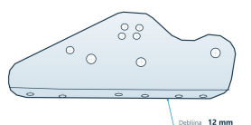
Lemken - Podešavajući nosač 4022566
